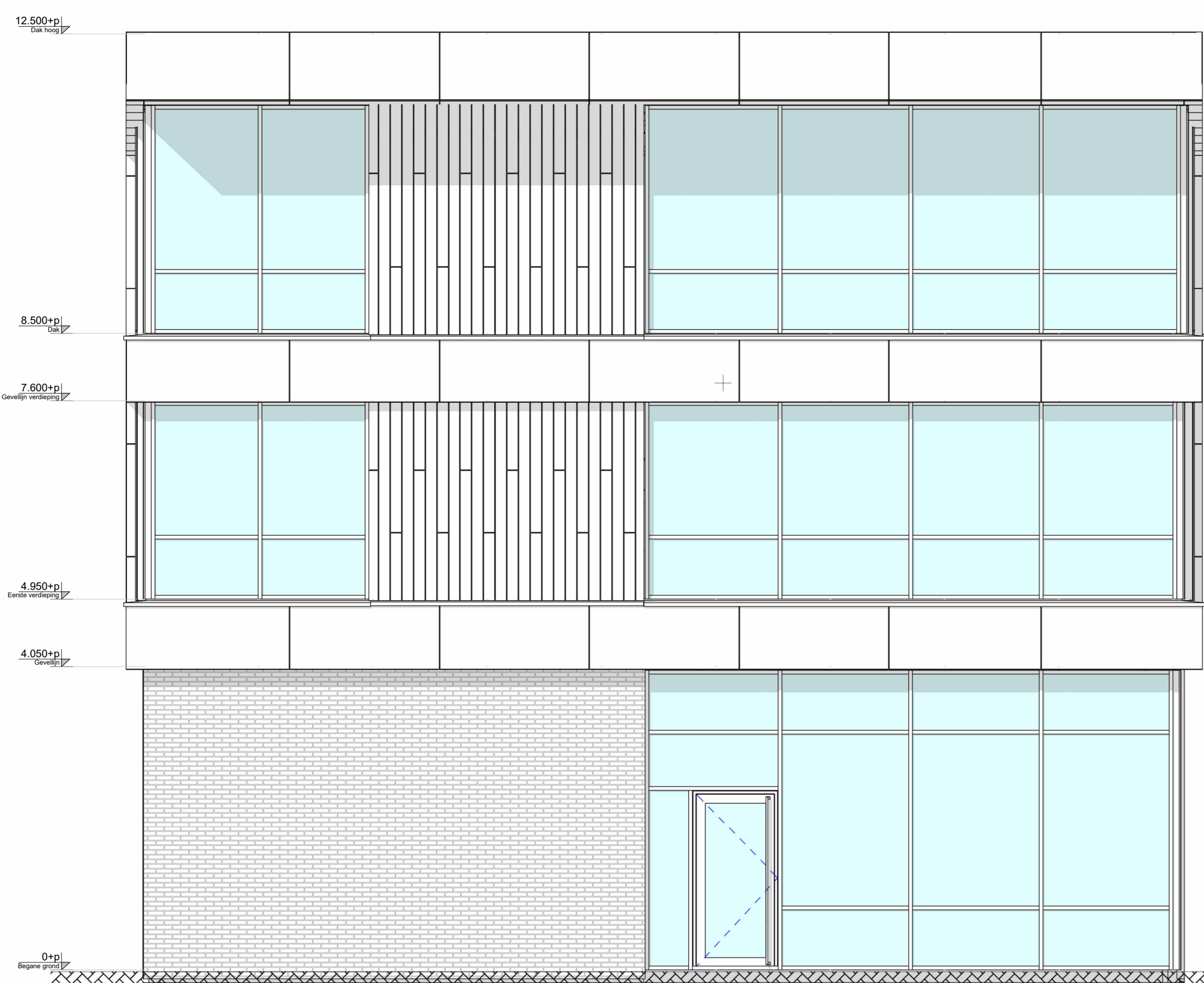
Voorgevel 1:50
