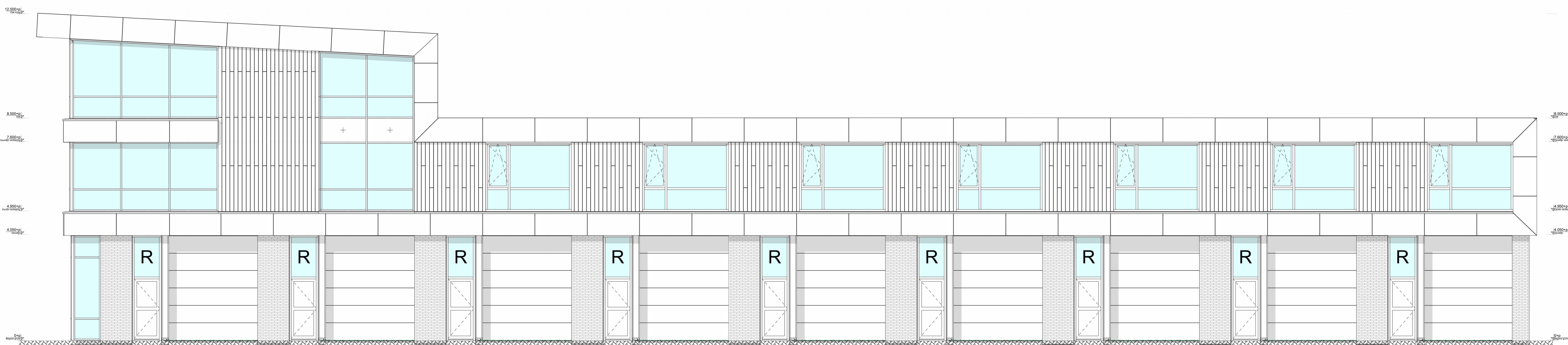
Binnengevel linkerblok 1:50
