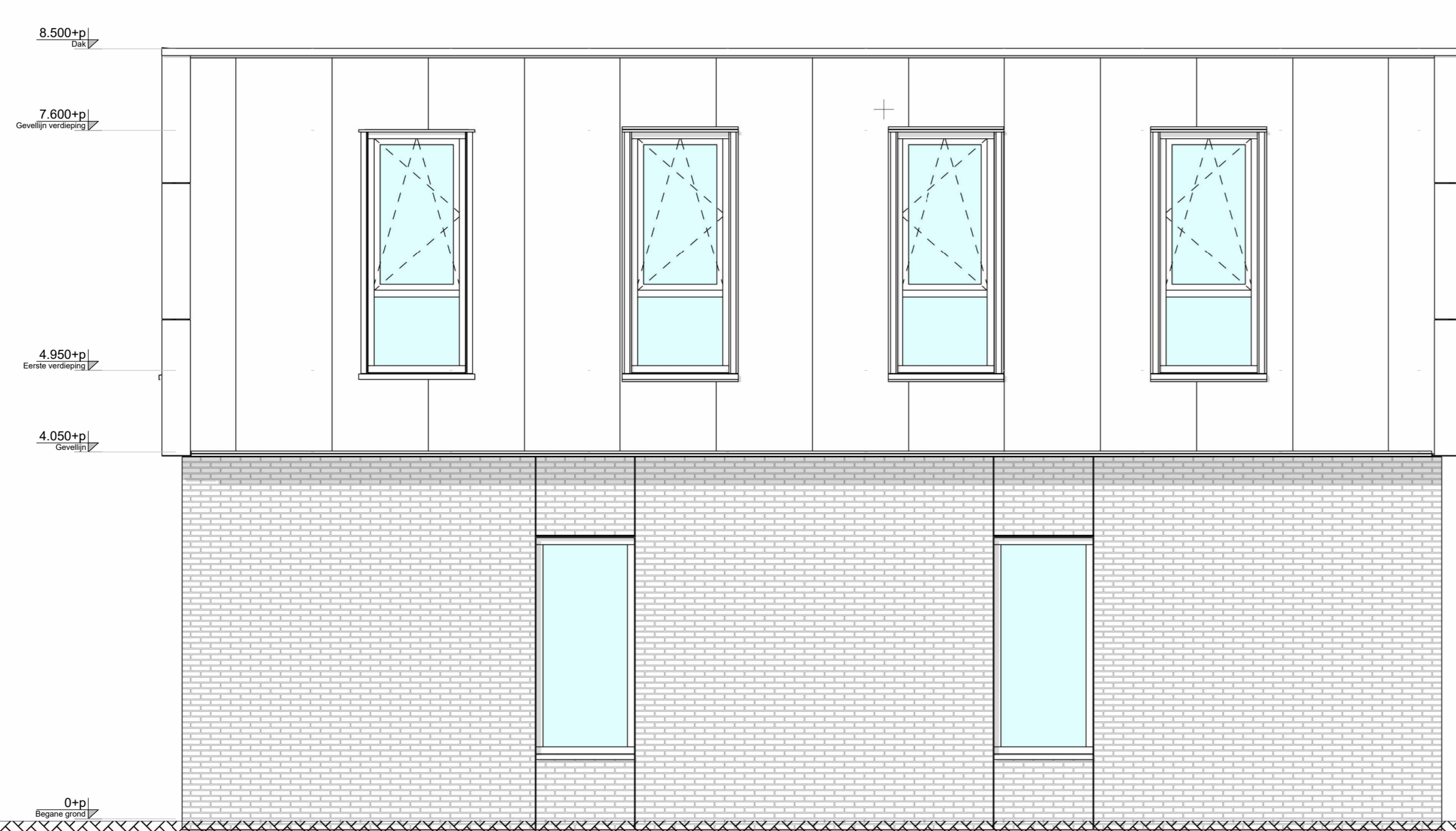
Achterevel 1:50
